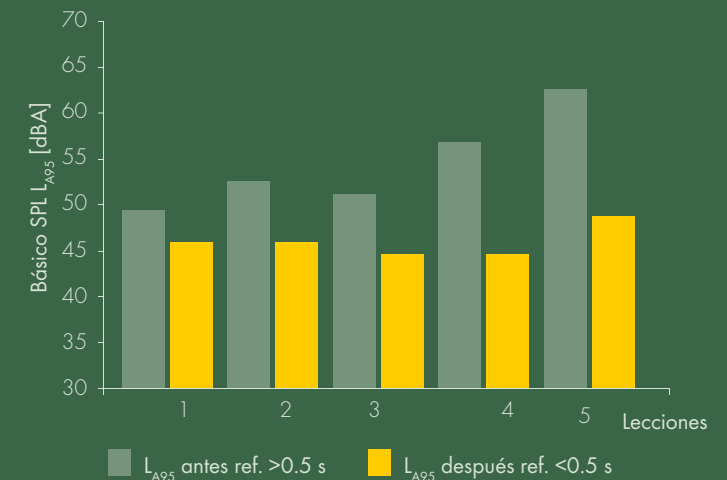
Aumento de los niveles sonoros de actividad ( L_{A95} ) antes y después de las reformas
