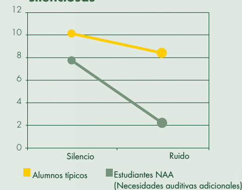
Puntuaciones de lectura en condiciones ruidosas frente a silenciosas
