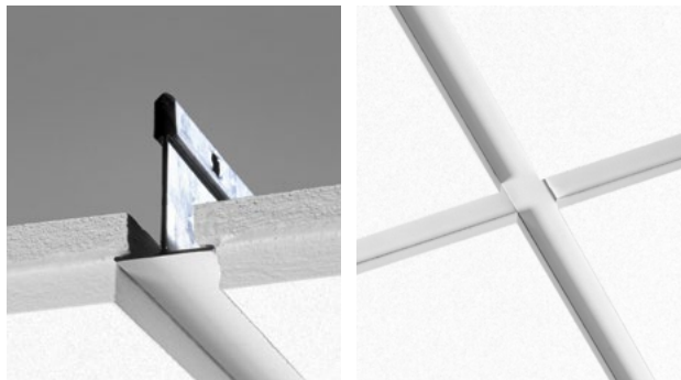
Pykäläreuna alaslaskettu lista-asennus, helposti avattavissa
