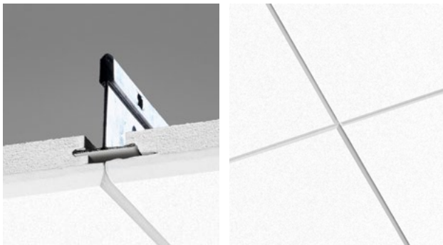
Viistetty reuna alaslaskettu symmetrinen piilolista-asennus, avattavissa
