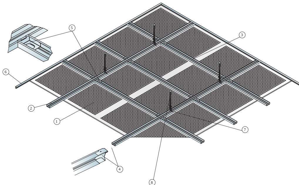
Asennuskuva (M608) Gyptone BIG Quattro, 2400x1200, alaslaskettu asennus 1-tasoisella GK-järjestelmällä
